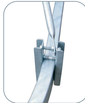
Ancoraggio tirante colonna anteriore Front column tie rod anchoring Attelage tirant colonne avant Vorgespannter Zuganker vordere Säule
