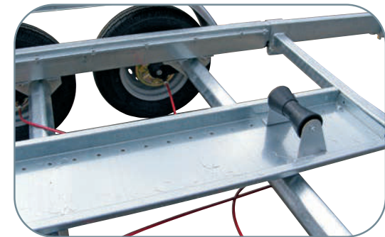
Appoggio deriva con battuta registrabile Drift support with adjustable stop Appui dérive avec butée ajustable Auflage für Kielschwert mit verstellbarem Anschlag
